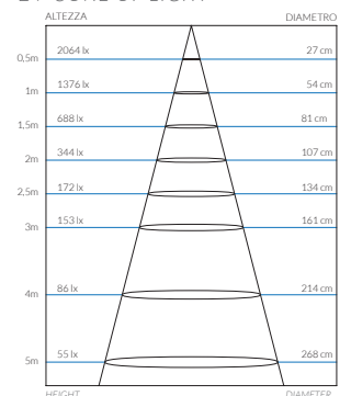
CONO DI LUCE 24° 24° CONE OF LIGHT
