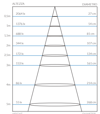
CONO DI LUCE 24° 24° CONE OF LIGHT
