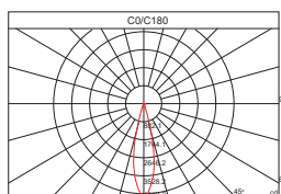
CURVA FOTOMETRICA
