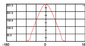
CURVA FOTOMETRICA
