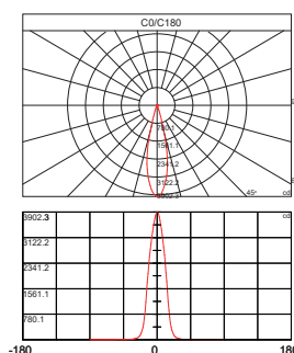
CURVA FOTOMETRICA
